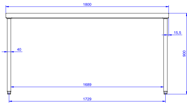
Front aanzicht
